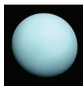
Urano
