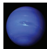
Neptuno
