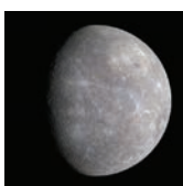
Mercurio
